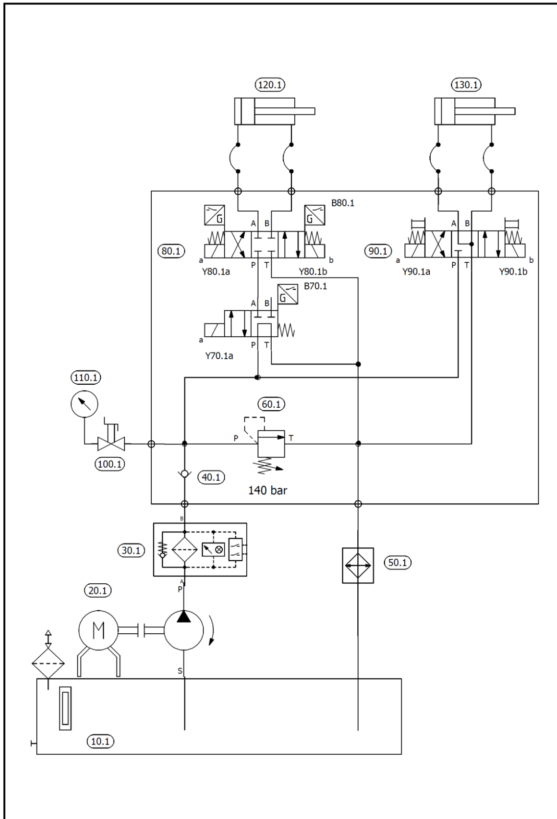
Figura 82: Circuito hidráulico
