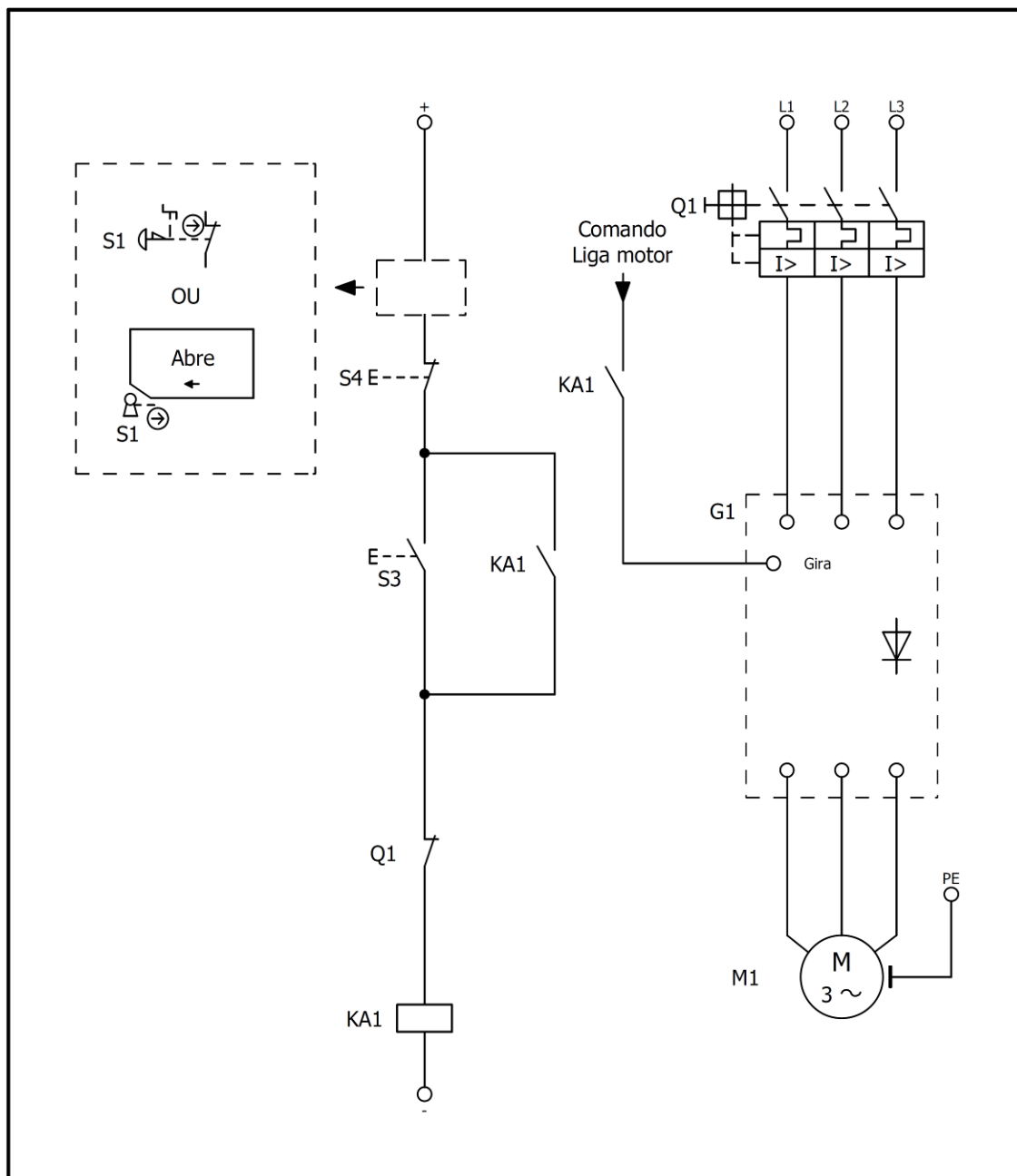
Figura 26: Circuito elétrico
