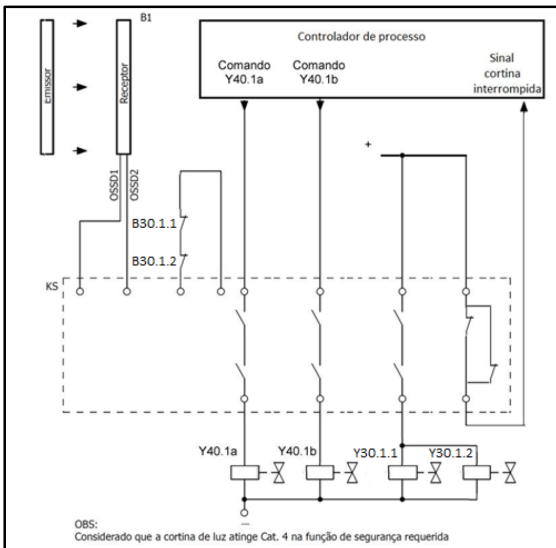
Figura 100: Circuito elétrico
