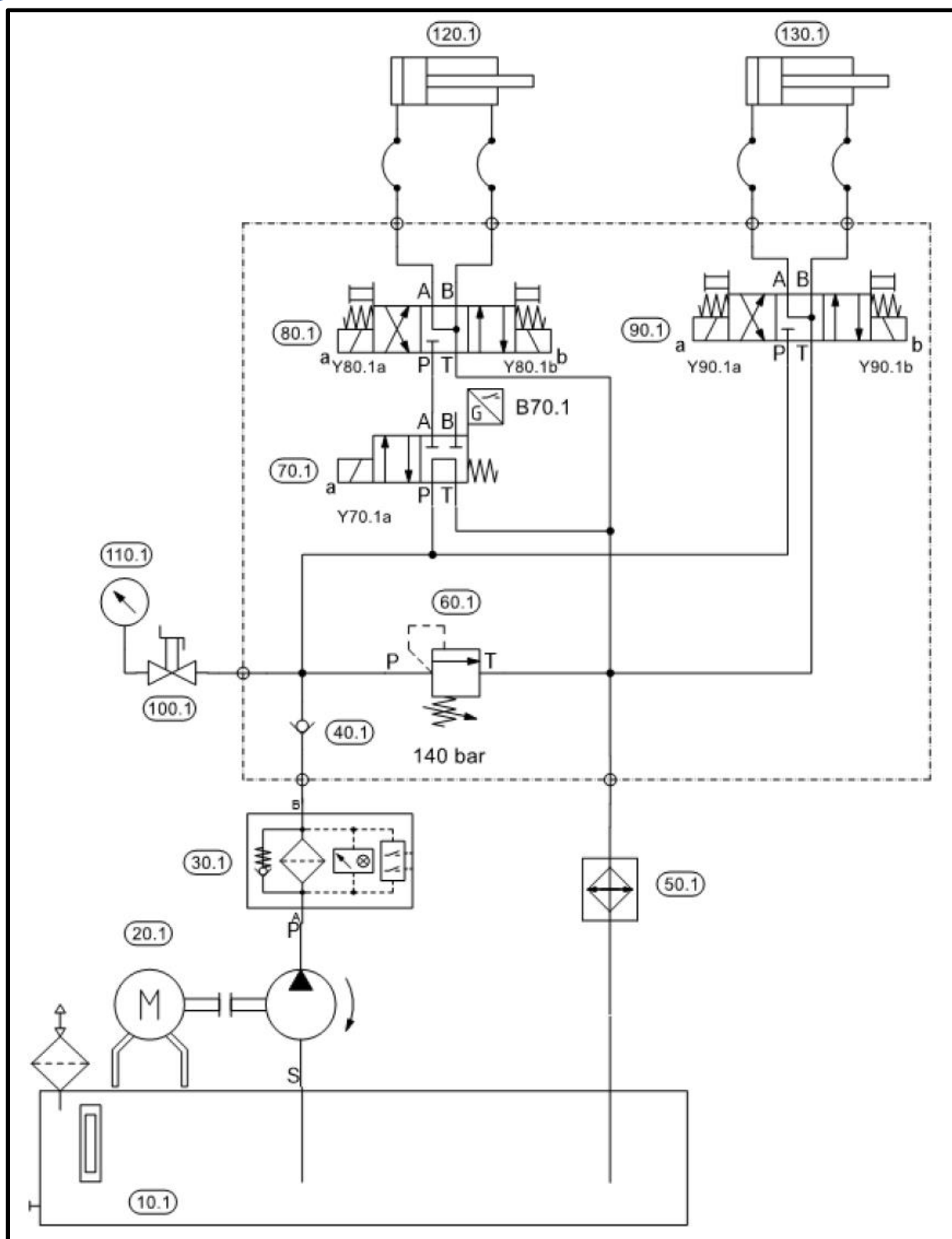
Figura 103: Circuito hidráulico
